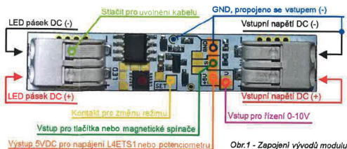
Obr.1 - Zapojení vývodů modulu
