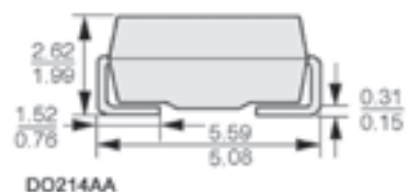
DO214AA
