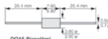
DO15 Bipolární
